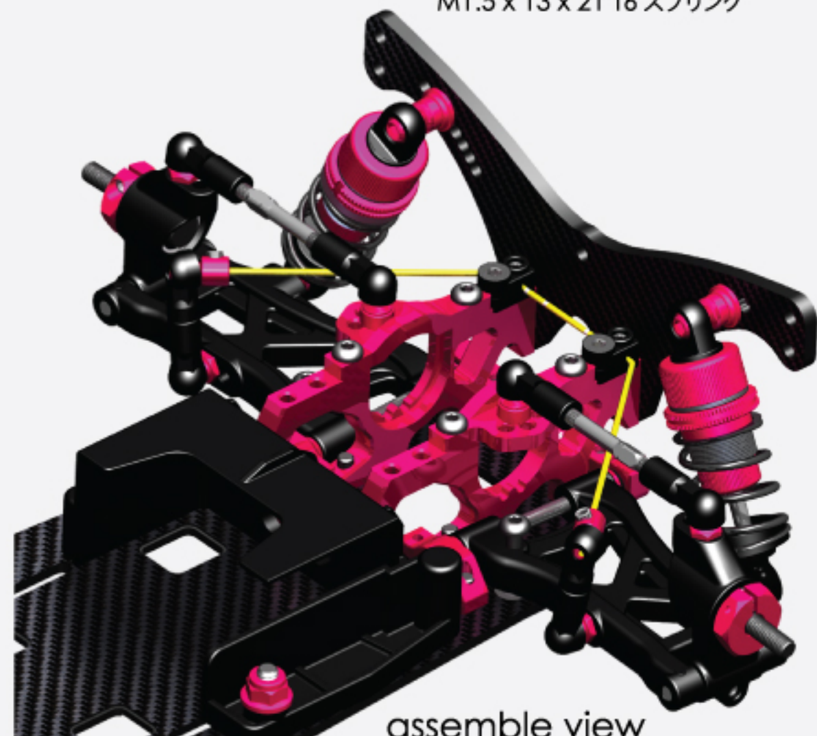
Rear Oil Shock / リア・オイルショック M1.5 x 13 x 21 T6 Spring M1.5 x 13 x 21 T6 スプリング
