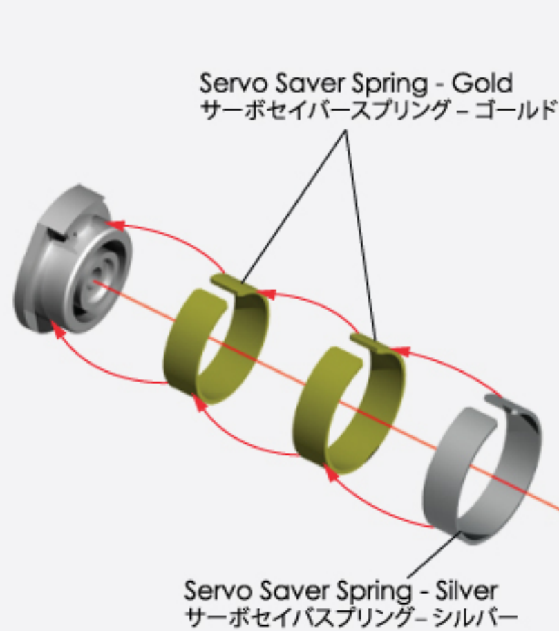
Servo Saver - SANWA, JR ACOMS, KO サーボセイバー - SANWA, JR ACOMS, KO
