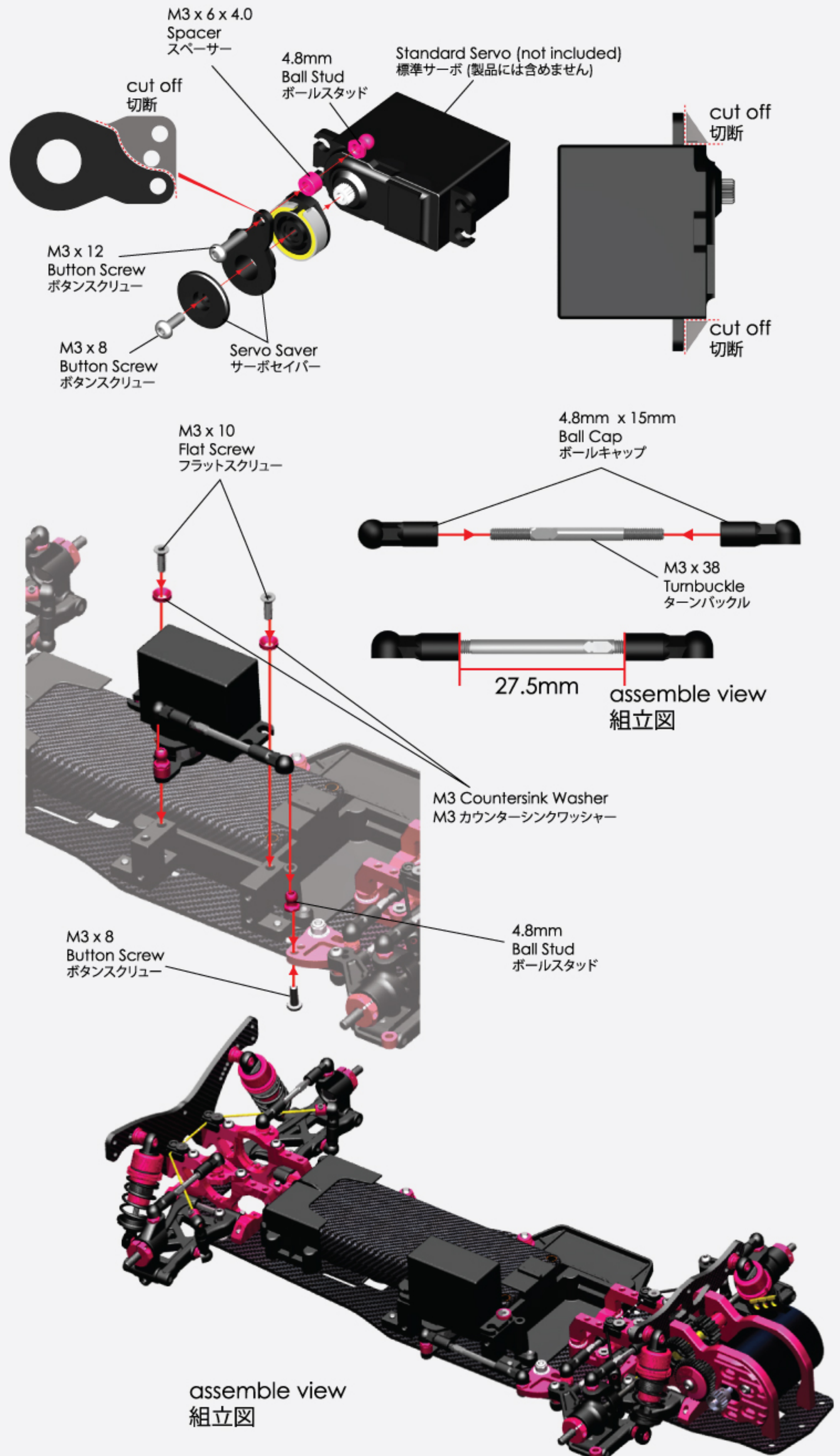
M3 x 10 Flat Screw (2) M3 x 10 フラットスクリュー (2)
