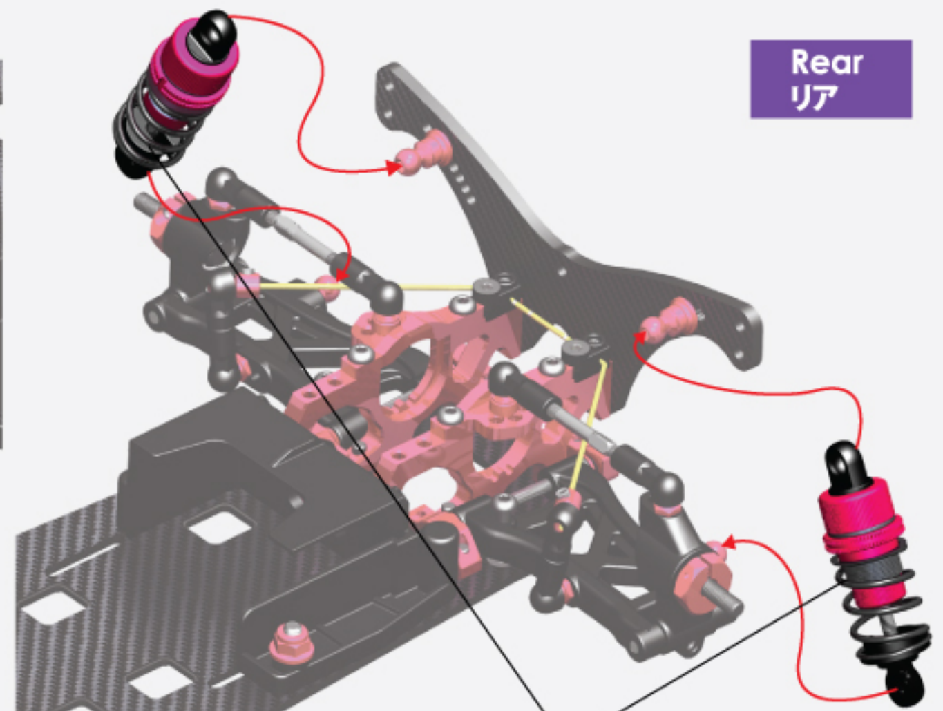
Rear Oil Shock / リア・オイルショック M1.5 x 13 x 21 T6 Spring M1.5 x 13 x 21 T6 スプリング
