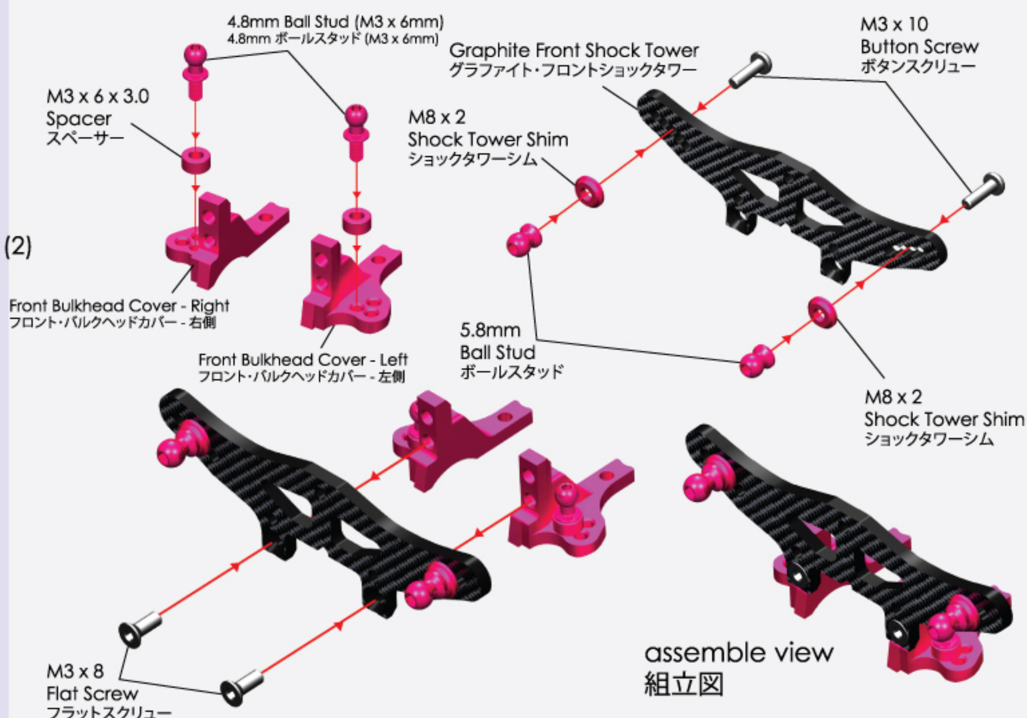
assembly view 組立図
