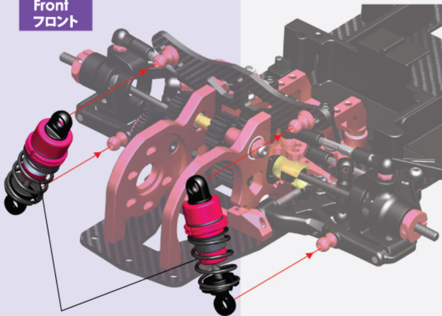
Front Oil Shock / フロント・オイルショック M1.5 x 13 x 21 T5.5 Spring M1.5 x 13 x 21 T5.5 スプリング
