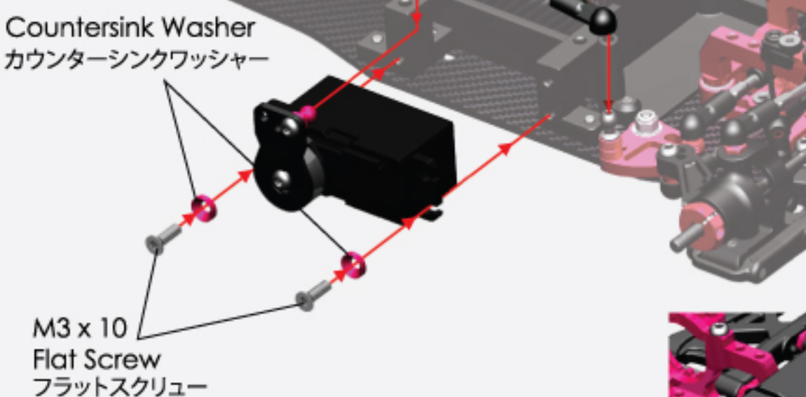
M3 x 10 Flat Screw (2) M3 x 10 フラットスクリュー (2)
